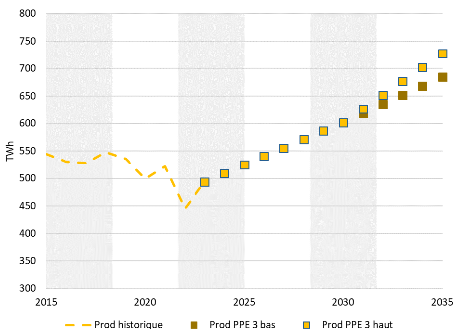
Figure 25 Projection de la production d'électricité à 2030 et 2035 (Source : Modélisations DGEC)
