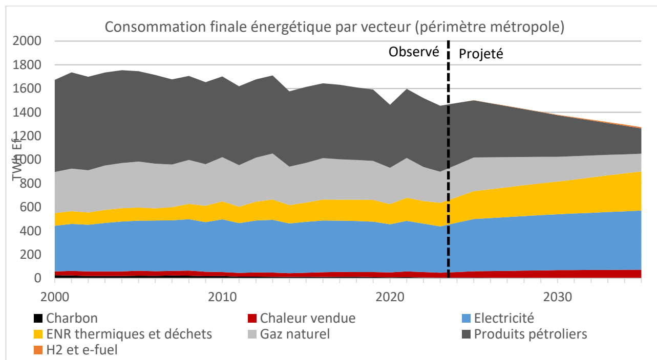
Figure 3 Evolution du mix énergétique réel (2000-2023) et projection des consommations finales énergétiques jusqu'en 2035 (SDES, mai 2024 ; Modélisation DGEC, hors soutes internationales)
