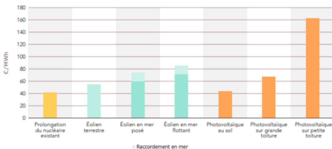
Figure 32 Comparaison des coûts complets annualisés (OPEX et annuités dues) pour les différentes capacités en exploitation à l'horizon 2030 dans la moyenne des six scénarios de mix étudiés dans Futurs énergétiques 2050 (p. 577, chiffres en €2020), hors coûts induits pour le système électrique
