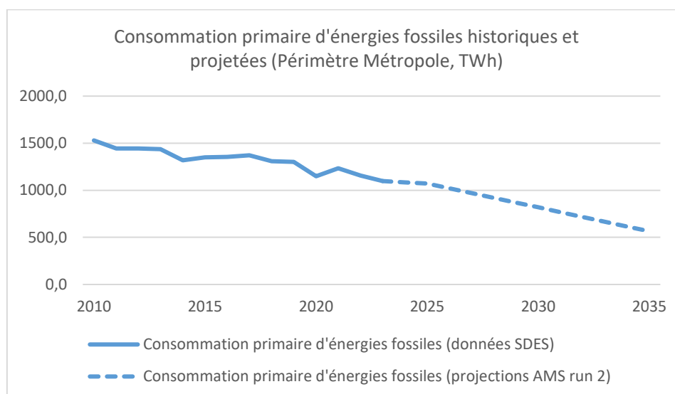
Figure 10. Consommation primaire d'énergies fossiles à usages énergétiques et non-énergétiques - Evolution passée (2010-2022) et projetée (2023-2035)
