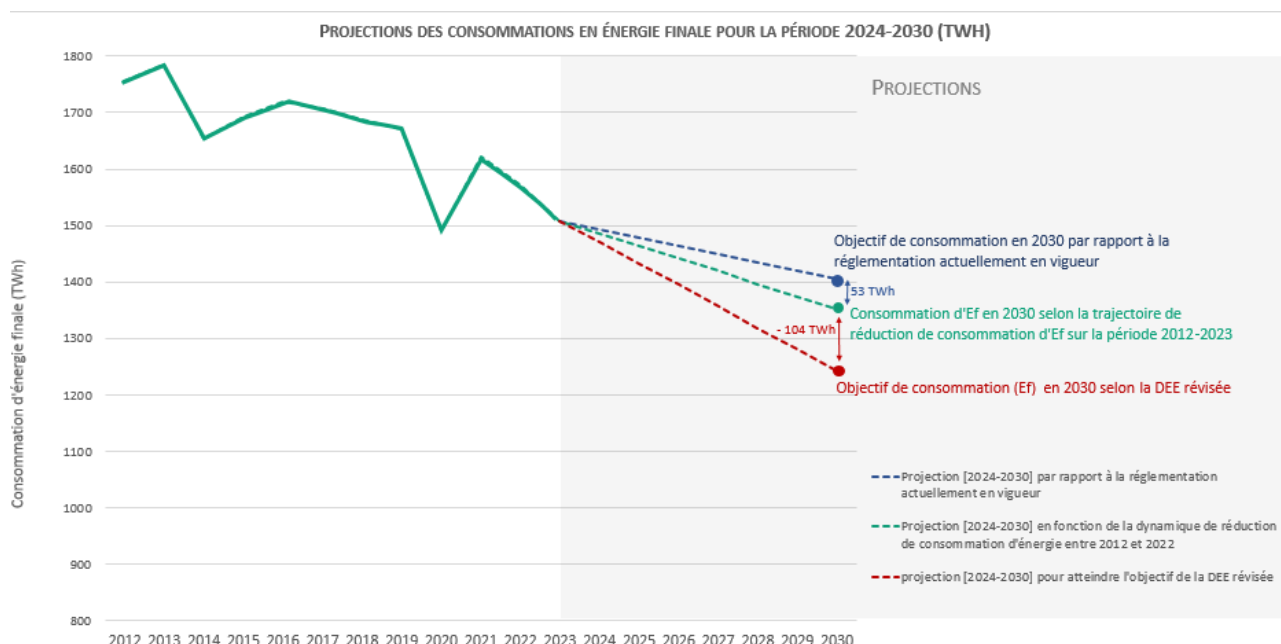
Figure 8. Projection des consommations en énergie finale à l'horizon 2030 (Modélisation DGEC sur la base des données du SDES 34 )
