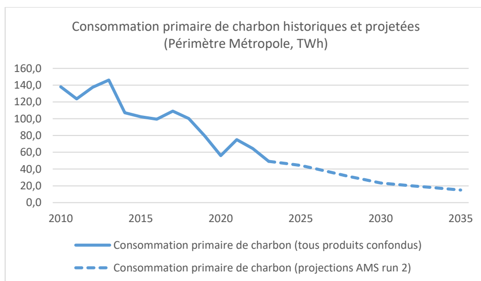
Figure 13. Consommation primaire de charbon historique et projetée
