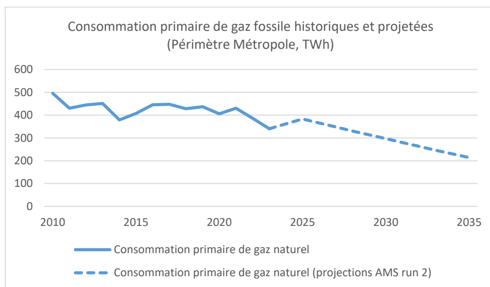
Figure 17. Consommation primaire de gaz naturel historiques et projetées
