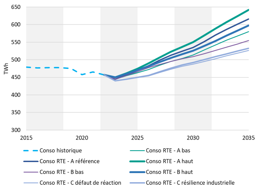
Figure 24. Projection de la consommation d'électricité à 2030 et 2035 (Source : RTE)
