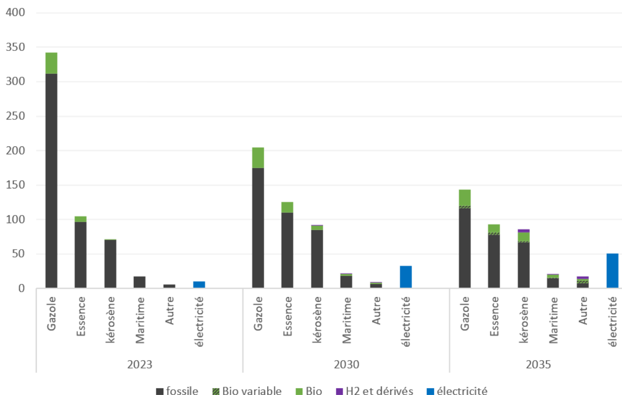
Figure 21. Evolution de la consommation d'énergie des transports (en TWh). Les données de consommation de 2020 et 2021 étant affectées par la crise COVID, l'année 2019 est retenue comme référence
